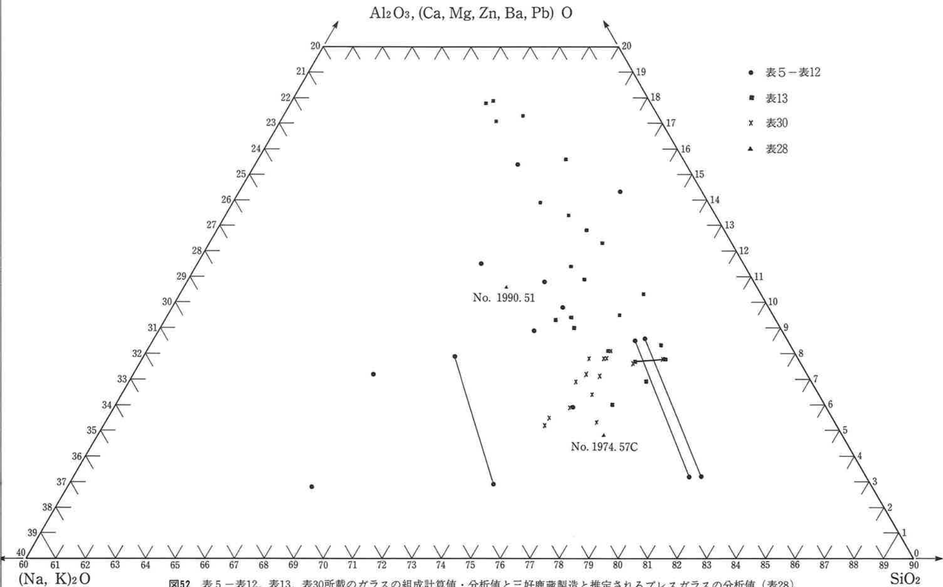
図52 表5-表12, 表13, 表30所載のガラスの組成計算値・分析値と三好鹿蔵製造と推定されるプレスガラスの分析値(表28)。
