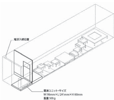
図 13. 電源ユニットの配置計画
